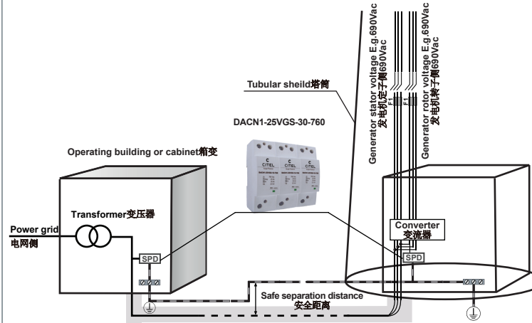
Fig. Double-fed induction asynchronous generator (DFIG) application 图. 异步双馈发电机 (DFIG) 应用案例
