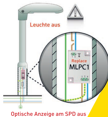
Bild 9: Überspannungsschutz defekt
