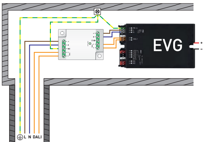
Installation MLPC(H*)1 mit DALI für Schutzklasse I
