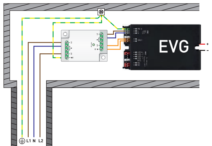
Installation MLPC1-2L zum Schutz für 2 (Steuer-) Phasen für Schutzklasse I
