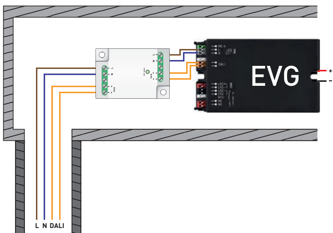
Installation MLPC(H*)2 mit DALI für Schutzklasse II
