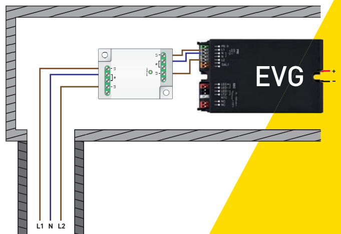
Installation MLPC2-2L zum Schutz für 2 (Steuer-) Phasen für Schutzklasse II
